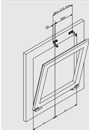
Apertura vasistas: Tracciare con la matita la mezzeria "X" del serramento.
