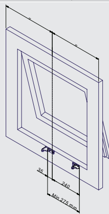
Верхнеподвесное окно, открытие наружу С помощью карандаша отметьте среднюю точку «Х» на оконной раме
