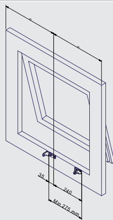
Apertura a sporgere: Tracciare con la matita la mezzeria "X" del serramento.
