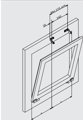
Нижнеподвесное окно, открытие внутрь С помощью карандаша отметьте среднюю точку «Х» на оконной раме.
